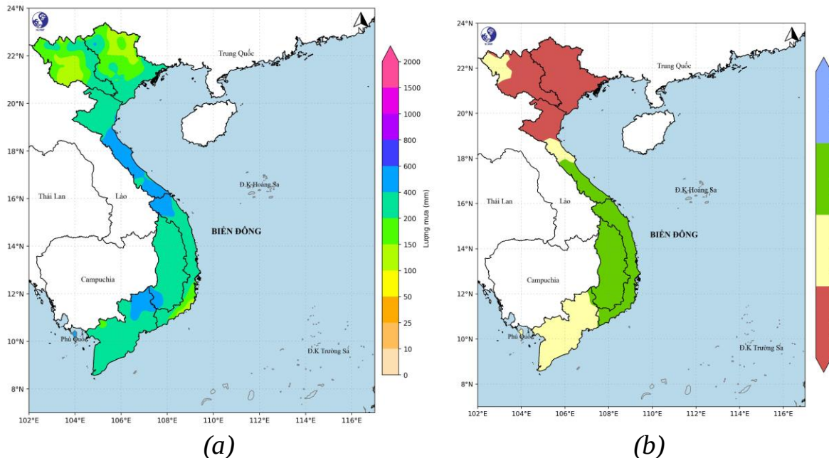
Hình 4: (a) Tổng lượng mưa (mm) TBNN tháng 9; (b) Dự báo xu thế lượng mưa tháng 9/2026
