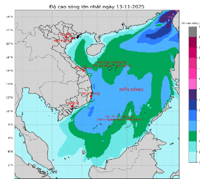
Hình 2. Bản đồ dự báo độ cao sóng
