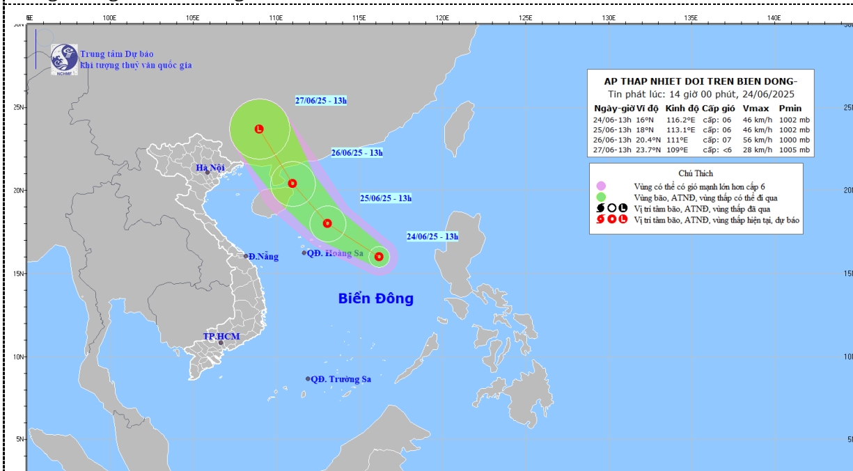
Hình1. Bản đồ dự báo quỹ đạo và cường độ áp thấp nhiệt đới lúc 14h00 ngày 24/6/2025
