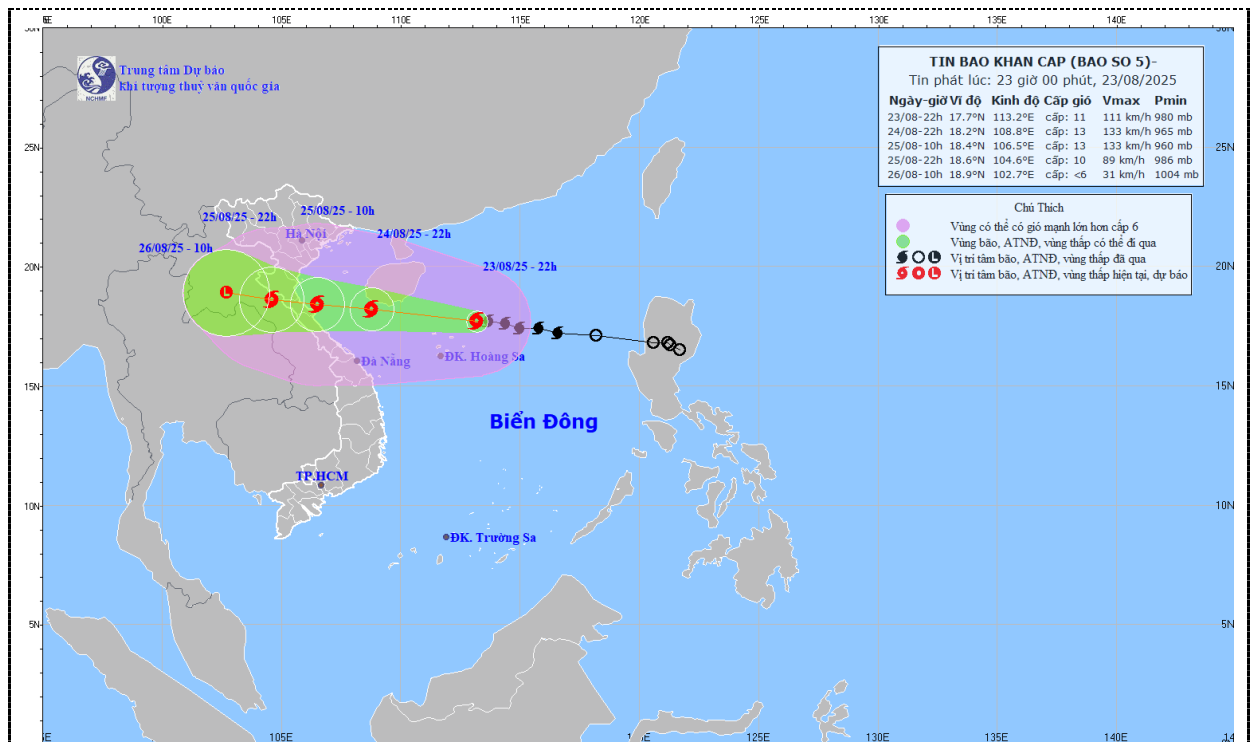
Hình 1. Bản đồ dự báo quỹ đạo và cường độ bão số 5 phát lúc 23h00 ngày 23/8/2025
