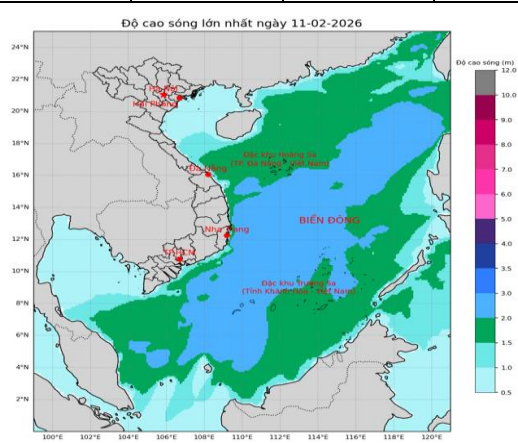
Hình 2. Bản đồ dự báo độ cao sóng
