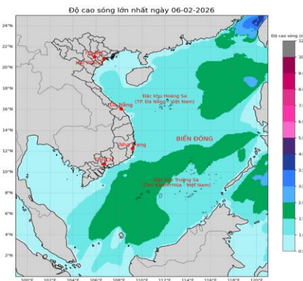
Hình 2. Bản đồ dự báo độ cao sóng
