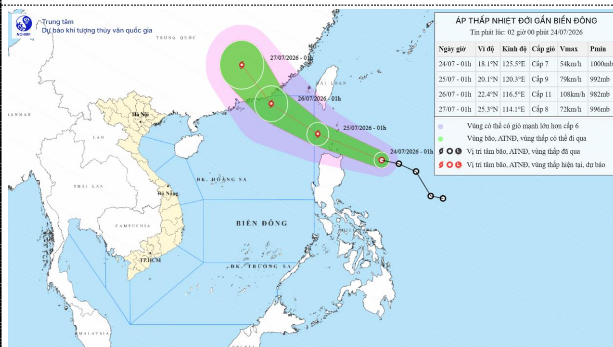
Hình1. Bản đồ dự báo quỹ đạo và cường độ áp thấp nhiệt đới phát lúc 02h00 ngày 24/7/2026
