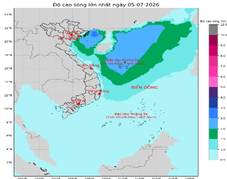
Hình 2. Bản đồ dự báo độ cao sóng
