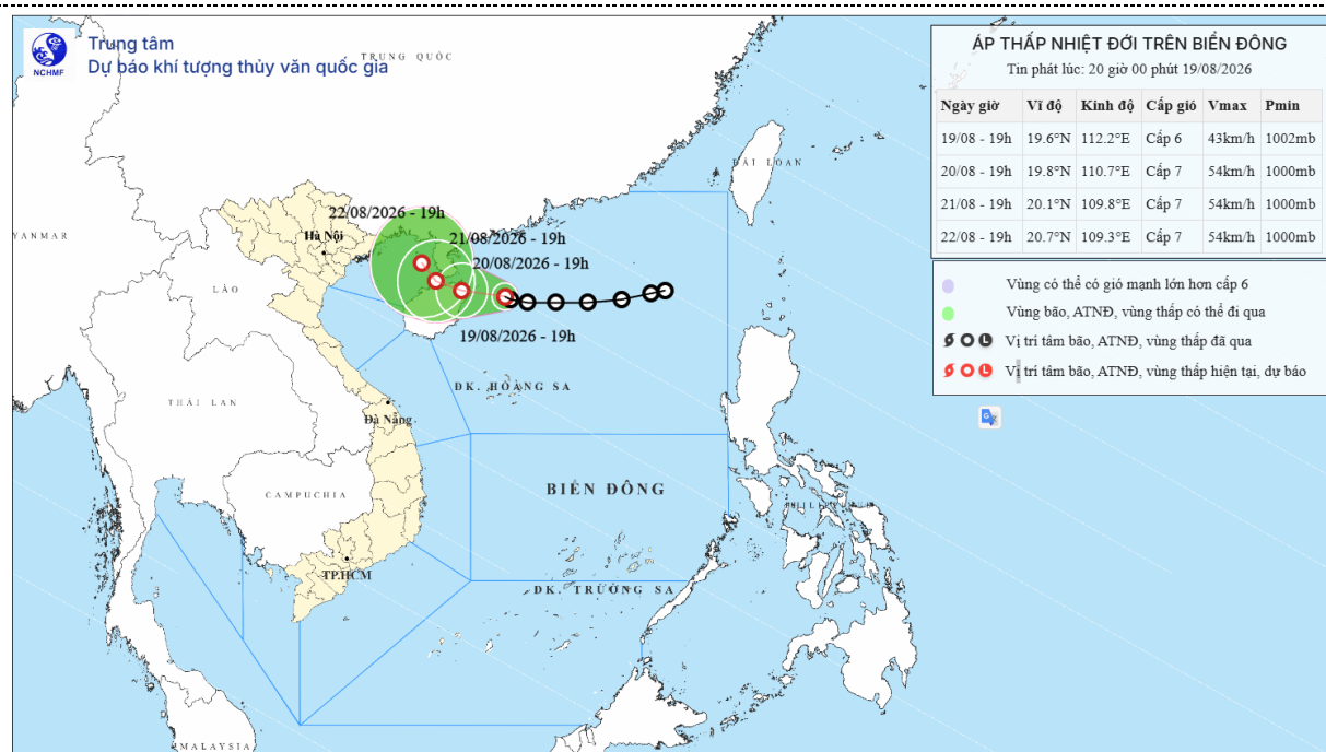
Hình 1. Bản đồ dự báo quỹ đạo và cường độ áp thấp nhiệt đới lúc 20h00 ngày 19/8/2026
