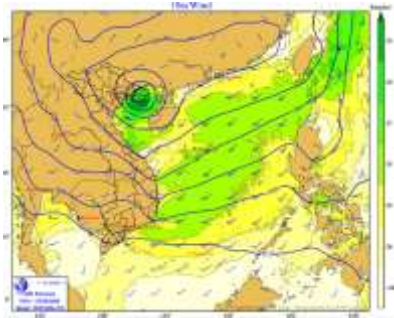
Hình 1. Bản đồ dự báo gió mạnh
