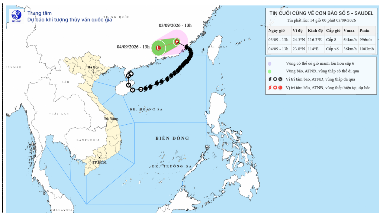
Hình 1. Bản đồ quỹ đạo bão số 5 tính đến 14h00 ngày 03/9/2026
